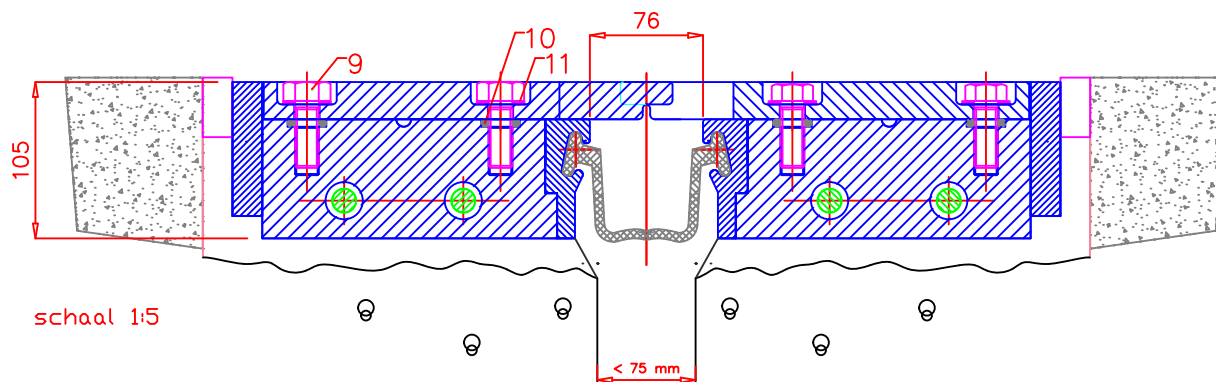
Doorsnede B-B gereed product incl. dekplaat
