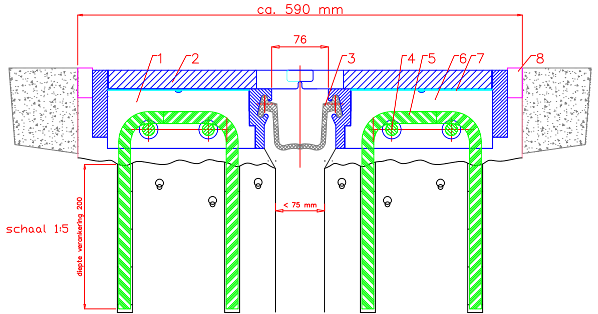
Doorsnede A-A gereed product incl. dekplaat
